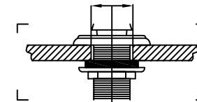
Trou d'installation douchette Ø30
