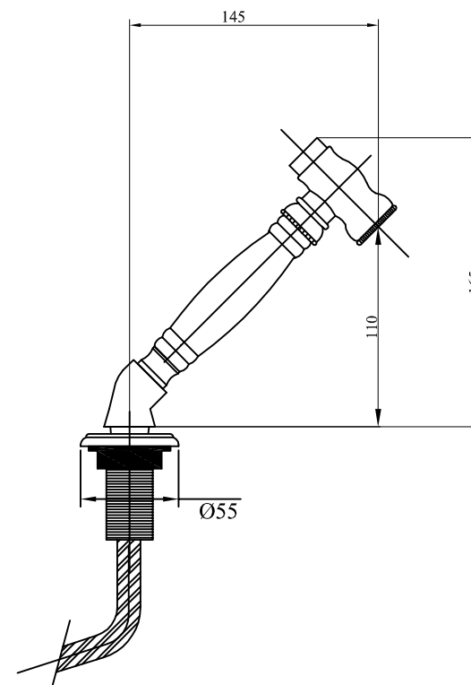
Trou d'installation corps Ø35
