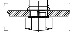
Trou d'installation corps Ø35
